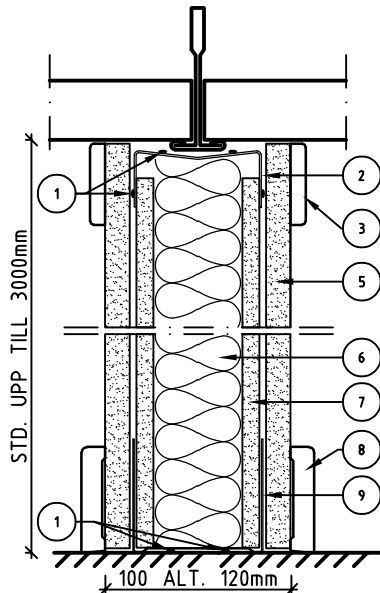
ALTERNATIV SEKTION B-B
