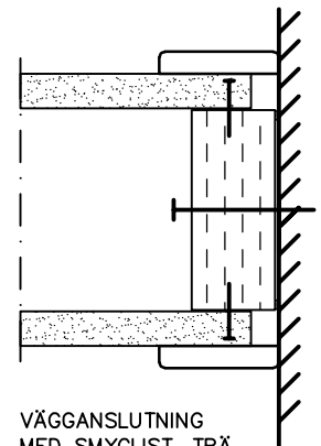
SEKTION C-C
