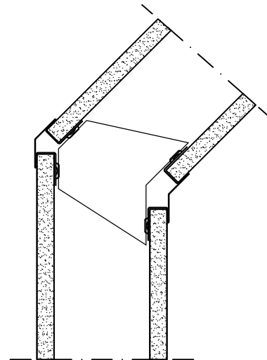
45° HÖRN
