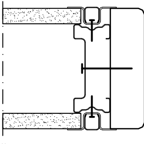
VÄGGAVSLUT MED INREDNINGSSKENA OCH DEKORLIST
