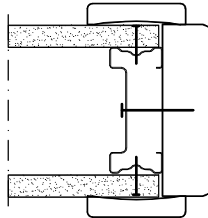
VÄGGAVSLUT MED FODER, TRÄ
