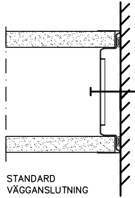
SEKTION C-C
