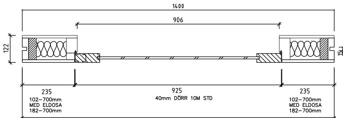
SEKTION ALTERNATIV B-B
