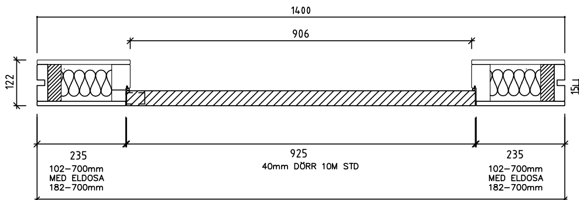
SEKTION ALTERNATIV B-B
